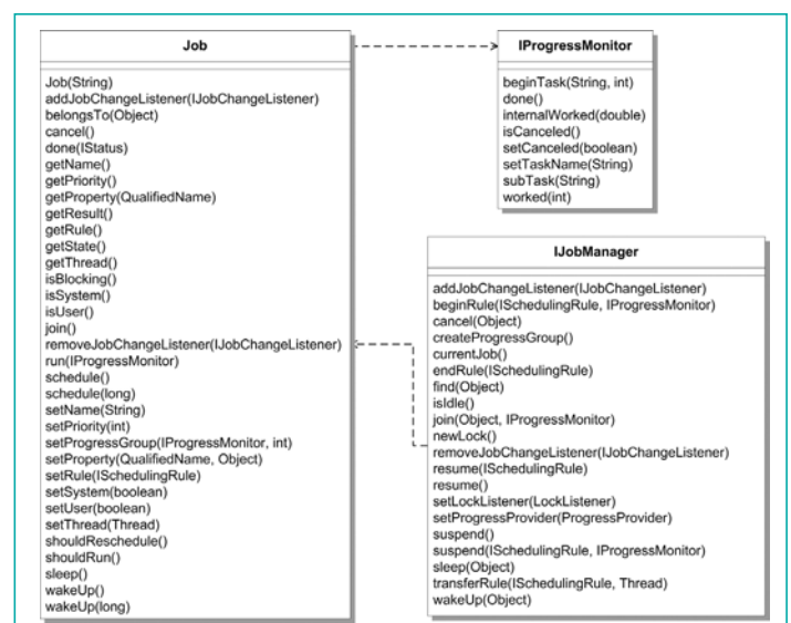
Abb. 1: Die wichtigsten Klassen des Job API
