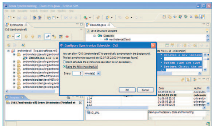
Abb. 4: Konfiguration der regelmäßigen CVS-Synchroni- sation
